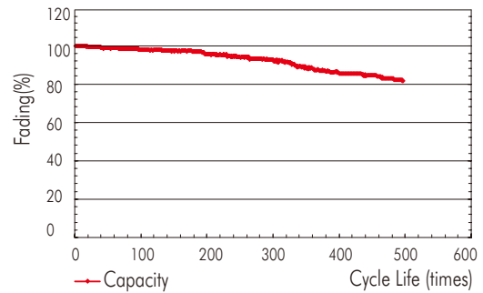
Cycle Life (23±2°C)
