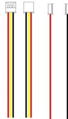
MOLEX87439-3P
